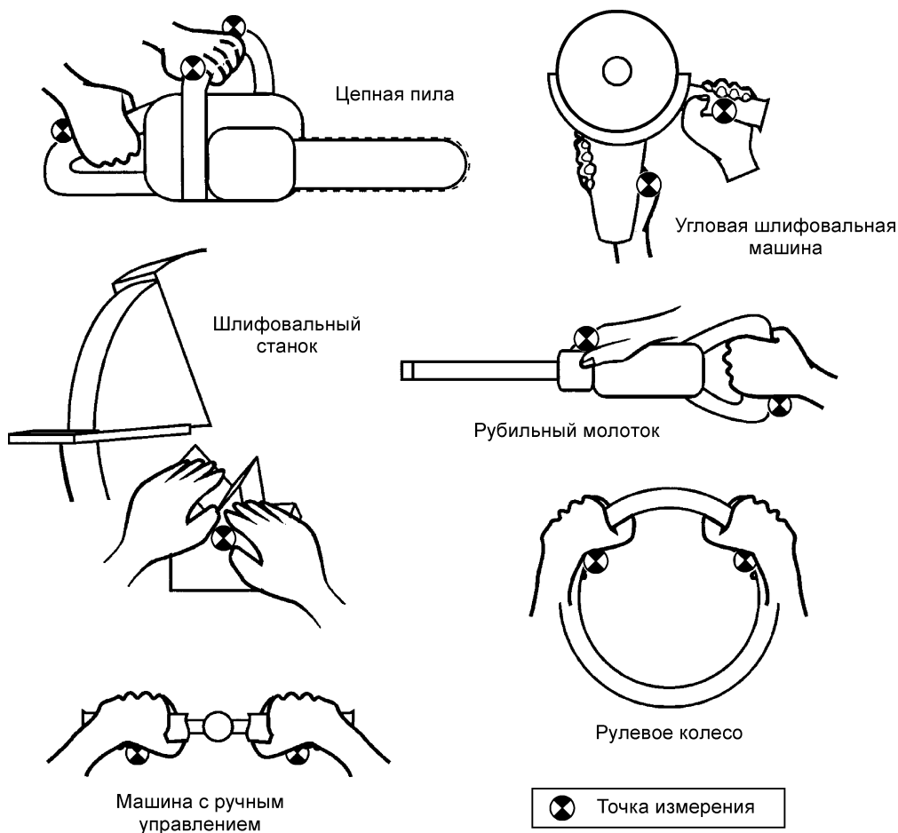
Рисунок А.1 — Примеры расположения точек измерения для типичных случаев воздействия локальной вибрации
